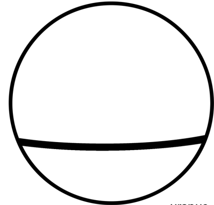
uranus
