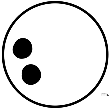
earth
