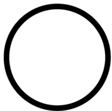
pluto
